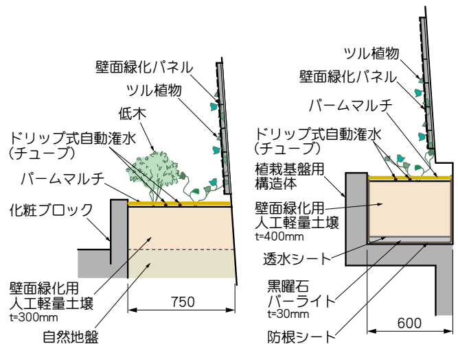
地上部 断面図
