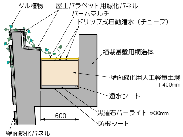
屋上部 標準断面図
